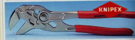
Tångnyckel KNIPEX . Drar med extremt hög presskraft och i varje position helt parallella käftar. Knappinställning och "spårskattsfunktion" vid nytt grepp. Särskilt lämplig för armaturer med kromad yta. Nr Gripv. Längd Pris 30-5610 35 mm 180 mm 398:- 30-5550 42 mm 250 mm 449:-
