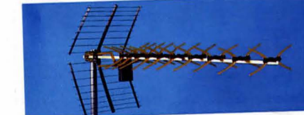
TV-antenn UHF 43 element. För kanal 21-65. Förstärkning 13 dB. Anslutning för koaxialkabel (75 ohm). Mastfäste. Längd 119 cm. 42-209 ..... Pr st 198:- ..... 10 st 1795:-
