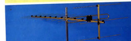
TV-antenn VHF 14 element. För kanal 5-12. Förstärkning 10,5 dB. Anslutning för koaxialkabel (75 ohm) eller bandkabel (300 ohm). Mastfäste. Längd 202 cm. 42-168 ..... 395:-
