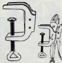
Bordshållare för 10" svetsstäng. Max bordstjocklek 65 mm. 30-5849 ..... 39:00
