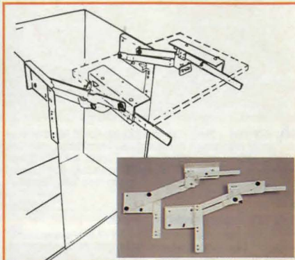
Köksmaskinslyft Endast de fjädrande beslagsdelarna. Hyllplan ingår ej. 41-2310..... 249:-
