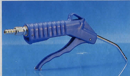
Blåspistol av plast med ventil och 1/4" slanganslutning. 30-4545 ..... 39:--
