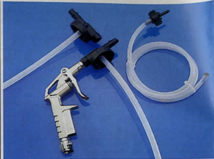
Sprutpistol för rostskyddsolja och karoskydd i 1-liters förpackning med gånganslutning. Levereras med två utbytbara anslutningsmunstycken samt 1 m slang med hålrumsmunstycke. 30-4840 ..... 119:--
