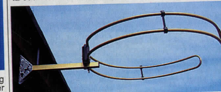
FM-antenn för radio. Rundmottagande. En utmärkt antenn för att ta emot flera FM-stationer som ligger geografiskt på olika ställen. Anslutning för 75 ohms koaxialkabel eller bandkabel. Väggfäste. Diameter 55 cm. 42-4009 ..... 198:—
