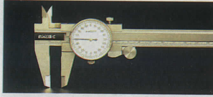
Skjutmått med mätur. Mätlängd 150 mm, avläsning 0,02 mm. Mattförokromad mätstång, skjutmåttet är av rostfritt stål. Skänkel längd 40 mm. Lev. i träetui. 30-3438 ..... 319:—
