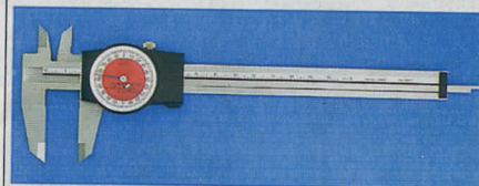
Skjutmått med klocka , (diam. 32 mm), roterande ring för nollställning. Härdade mätskänklar. Mätlängd 150 mm, nomie 0,02 mm. DIN 862. Levereras i träetui. 30-4720 ..... 595:--
