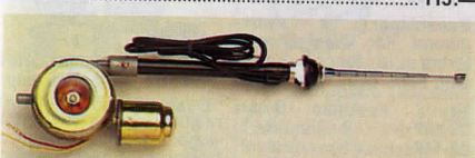
Bilantenn, heliomatic. 5 sektioner, längd 1 m. Antennen är i nedskjutet läge låst och skyddas på så sätt från att brytas eller vandaliseras. Inkopplas så att antennen skjuts ut eller in vid eller avstängning av bilstereoapparater, som har uttag för automatisk bilantenn. 12 V. Vikt 1 kg. Inbyggnadsmått: 32 x 10 x 6 cm. 32-3708 ..... 345:—
