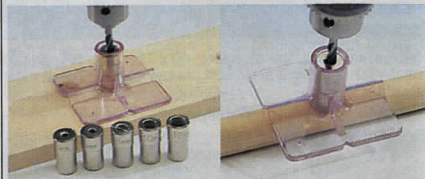
Borrguide . Ny modell för enkel borring i 90°, på kanter, runda material m.m. Sex styrhylsor för 4, 5, 6, 8, 10 och 12 mm borrar medföljer. 20-4828 ..... 69:--
