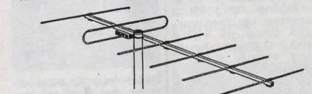
TV-antenn VHF 7 element. För kanal 5-12. Ansl.dosa för 300/75 ohm. Förstärkning 9 dB. Lev. med både mastfäste och väggfäste. Längd 120 cm. 42-970 ..... 260:—
