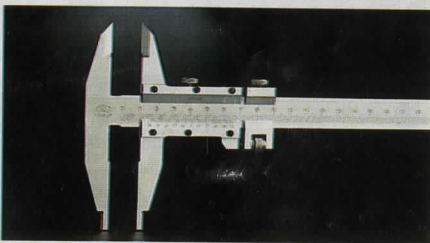
Verkstads-skjutmått med mattförokromad skala. Graderad i mm och med nonie för 1/20 mm. Mätlängd 300 mm. Skjutmåttet har fininställning och skänklar för invändigt mätning. 30-4046 ..... 319:—
