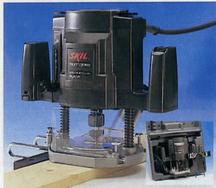
Handöverfräs SKIL 1835 U. Kraftig maskin med spindellås för snabbt bitsbyte. Vridbart anslag för förinställning av tre olika fräsdjup. Tomgångsvarv 25.000/min. Ineffekt 800 W. Vikt 3,2 kg. Lev. med spännhylsor för 6 och 8 mm skaft, sidoanslag, nycklar samt dammsugsadapter. Förpackat i kraftig transportväska. 40-4192 ..... 1598:—
