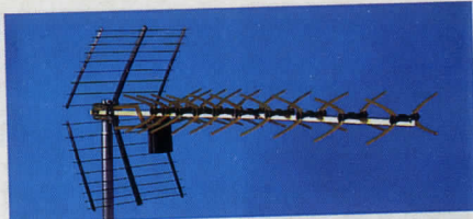
TV-antenn UHF. 43 element, kanal 21-65. Förstärkning 13 dB. Anslutning för koaxialkabel (75 ohm). Mastfäste. Längd 119 cm. 42-209 ..... 225:—
