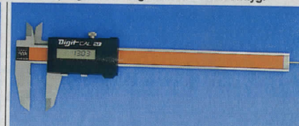
Digitalt skjutmått , mätlängd 150 mm eller 6 tum. Omsättningsbar mellan millimeter och tum. Nollställning på hela skalan. Digital utgång. Noggrannhet 0,01 mm. DIN 862. Levereras i träetui. 30-4721 ..... 1150:--
