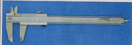
Skjutmått , härdat, med mattförkromad skala. Mätlängd 150 mm, nomie 0,02 mm. DIN 862. Levereras i träetui. 20-4719 ..... 495:--
