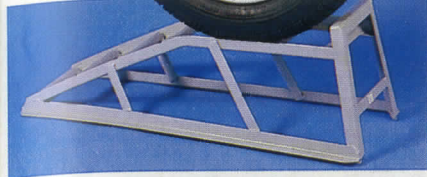
Uppkörningsramp för personbilar. Mått 850 x 250 x 230 mm. Tillåten last/rampar-tjänstevikt 1,5 ton. 40-3785 ..... Pr par 239:—
