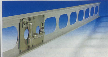
Vattenpass , TOTTMAR, 180 cm. Stege av heldragen lättmetallprofil. Justerbart våg- och lodbeslag med eterfyllda libeller. Bredd 107 mm. Vikt 2,5 kg. 40-3155 ..... 859:--
