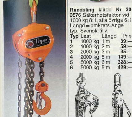
Lyftblock i mycket kraftigt utförande. Lättdragen kedja. Helt inkapslad broms och växelhuss. Vridbara krokar. Max. belastning 1000 kg. Lyfthöjd 2,5 m. Minsta krokavstånd 325 mm. Vikt 13,5 kg. Godk. enl. ASS anvisningar. 40-3567 ..... 898:—
