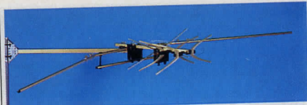
Kombi-antenn, 10 element. VHF kan.2 - 4, UHF kan. 21 - 68. Förstärkning VHF 3 dB, UHF 8,5 dB. Längd 44 cm. Anslutningsdosa för gemensam band eller koaxialkabel. Lev. med ställbart väggfäste. 42-238 ..... 265:—
