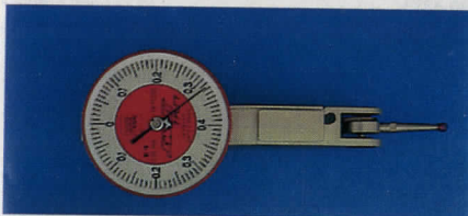
Vippindikator , diam. 28 mm. Noggrannhet 0,01 mm. Mätområde 0,8 mm, vippspetsens längd 12 mm. 30-4723 ..... 545:--
