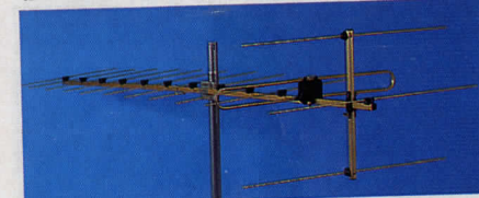
TV-antenn VHF 14 element. För kanal 5-12. Förstärkning 10,5 dB. Anslutning för koaxialkabel (75 ohm) eller bandkabel (300 ohm). Mastfäste. Längd 202 cm. 42-168 ..... 325:—
