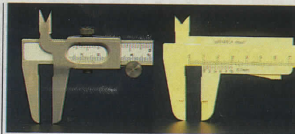
Skjutmått , av hög kvalitet med nonieskala, 120 mm. Användbart för ytter-, inner- och djupmått. Löparen förflyttas med friktionsrulle. 20-945 ..... 37:—
