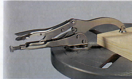
Materialhållare . Självslående med utlösningsarm. Oumbärligt hjälpmedel vid bearbetning av arbetsstycken med pelarbormaskin. Fästes vid bordet med 1/2" bult och öglemutter. Totallängd: 240 mm, max gripvidd: 65 mm. 30-4827 ..... 119:--
