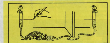
Slangvattenpass av genomskinlig graderad plast. För långa avstånd. Fästes på 1/2" slang och fylls med vatten för att mäta nivåskillnad. Lämplig slang 49-297. 30-4010 ..... 92:--
