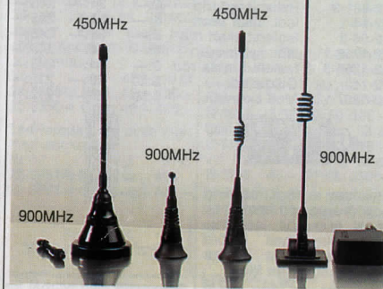
Mobiletelefonantenn med 2 st kvartsvågsspön av svart plastöverdragen stålwire för 450 och 900 MHz-bandet. Kraftigt magnetfot, diam. 6 cm. 3 m koaxialkabel med BNC anslutning. Lev. i praktiskt etui. Höjd med 900 MHz antenn 10 cm, 450 MHz 17 cm. 32-3902 ..... 395:—
