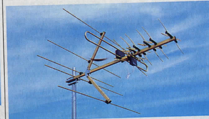
TV-antenn KOMBİ, 28 element. För både TV1 (kanal 5-12) och TV2 (kanal 21-69). Förstärkning 6,5 dB resp. 9 dB. Mastfäste. Anslutningsdosa för en gemensam bandkabel eller koaxialkabel. Längd 108 cm. 42-960 ..... 325:—
