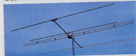
TV-antenn 4 element för kanal 2-4. Förstärkning 5,5 dB. Längd 178 cm. Anslutning för 75 ohms koaxialkabel eller bandkabel. Mastfäste. 42-4008 ..... 345:—
