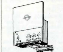
Antennförstärkare ASTRO KTS 50 med separat nätdel. Selektivbredbandsförstärkare för utomhusmontage. Lämplig för antennmast 50 mm Ø eller för väggmontage. För 75 ohms koaxialkabel. Förstärkning band FI-II, FIII 24 db, FIV-V 23 db. Brus 3,5-4,0 db. Nätdel för 220 V. S-märkt. 32-899 ..... 795:—
