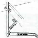
Väggfäste, justerbart 295-440 mm. Passar 1 1/2" maströr. tillv. av 35 x 5 mm galv. plattjärn. Lev. komplett med skruv. Utan maströr. 32-447 ..... 98:—
