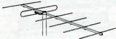
TV-antenn VHF 7 element. För kanal 5-12. Ansl.dosa för 300/75 ohm. Förstärkning 9 dB. Lev. med både mastfäste och väggfäste. Längd 120 cm. 42-970 ..... 215:—
