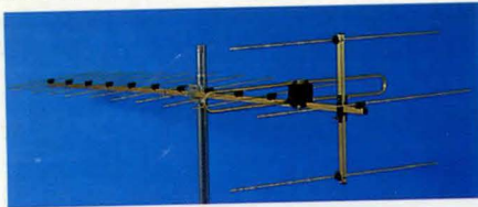
TV-antenn VHF 14 element. För kanal 5-12. Förstärkning 10,5 dB. Anslutning för koaxialkabel (75 ohm) eller bandkabel (300 ohm). Mastfäste. Längd 202 cm. 42-168 ..... 285:—
