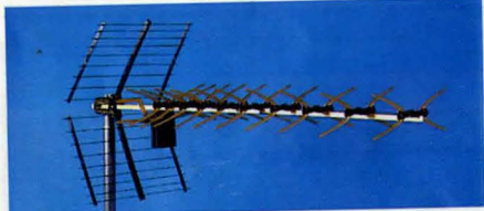
TV-antenn UHF. 43 element, kanal 21-65. Förstärkning 13 dB. Anslutning för koaxialkabel (75 ohm). Mastfäste. Längd 119 cm. 42-209 ..... 198:—
