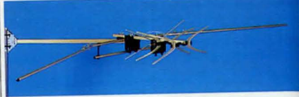
Kombi-antenn, 10 element. VHF kan.2 - 4, UHF kan. 21 - 68. Förstärkning VHF 3 dB, UHF 8,5 dB. Längd 44 cm. Anslutningsdosa för gemensam band eller koaxialkabel. Lev. med ställbart väggfäste. 42-238 ..... 235:—
