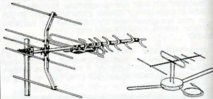
TV-antenn KOMBI, 28 element. För både TV1 (kanal 5-12) och TV2 (kanal 21-69). Förstärkning 6,5 dB resp. 9 dB. Mastfäste. Anslutningsdosa för en gemensam bandkabel eller koaxialkabel. Längd 108 cm. 42-960 ..... 279:—
