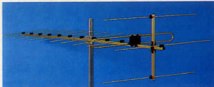
TV-antenn VHF 14 element. För kanal 5-12. Förstärkning 10,5 dB. Anslutning för koaxialkabel (75 ohm) eller bandkabel (300 ohm). Mastfäste längd 202 cm. Nr 42-168 ..... 254:—
