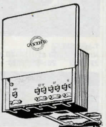
Antennförstärkare ASTRO KTS 50 med separat nätdel. Selektivbroadbandsförstärkare för utomhusmontage. Lämplig för antennmast 50 mm Ø eller för väggmontage. För 75 ohms koaxialkabel. Förstärkning band FI-II, FIII 24 db, FIV-V 23 db. Brus 3,5-4,0 db. Nätdel för 220 V. S-märkt. Nr 32-899 ..... 740:—
