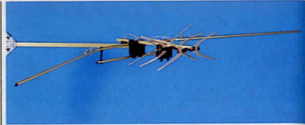
Kombi-antenn , 10 element. VHF kan.2 - 4, UHF kan. 21 - 68. Förstärkning VHF 3 dB, UHF 8,5 dB. Längd 44 cm. Anslutningsdosa för gemensam band eller koaxialkabel. Lev. med ställbart väggfäste. Nr 42-238 ..... 198:—
