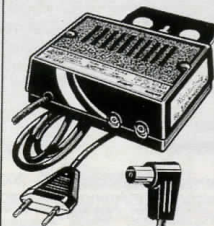
Antennförstärkare ASTRO. Bredbandsförstärkare för VHF, UHF och UKV. Förstärker antensignalen och ger därmed klarare bild, rek. för färg-TV. Förstärkning TV1 12 dB, TV2 10 dB. Koaxialanslutningar för in o. utgång. Uttag för 2 apparater. Lev. med monterad propp på ingång samt 2 st proppar för utgång. Anslutes till 220 V. S-märkt. Nr 32-718 ..... 398:—
