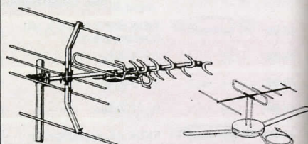
TV-antenn KOMBİ , 28 element. För både TV1 (kanal 5-12) och TV2 (kanal 21-69). Förstärkning 6,5 dB resp. 9 dB. Mastfäste. Anslutningsdosa för en gemensam bandkabel eller koaxialkabel. Längd 108 cm. Nr 42-960 ..... 265:—
