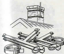
Skorstensfäste . Dubbelt fäste för 2" antennmast. Kraftig och gediget utfört och korrosionssäkrat helt varmgalvaniserat. Det är enkelt o. snabbt att montera och sitter säkert. Bandlängd 2 x 5 m. Nr 32-1069 ..... 98:—
