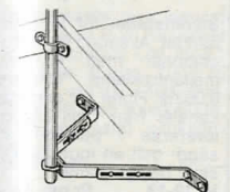
Väggfäste , justerbart 295-440 mm. Passar 1 1/2" maströr, tillv. av 35 x 5 mm galv. plattjärn. Lev. komplett med skruv. Utan maströr. Nr 32-447 ..... 90:—
