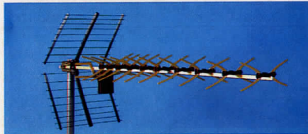
TV-antenn UHF . 43 element, kanal 21-65. Förstärkning 13 dB. Anslutning för koaxialkabel (75 ohm) eller bandkabel (300 ohm). Mastfäste längd 119 cm. Nr 42-209 ..... 198:—
