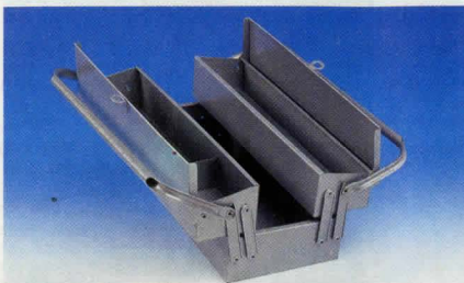
Verktyslåda av brännlackerad, kraftig plåt med rörhandtag. Består av tre sammansatta lådor, vikt ca 2,5 kg. Yttre mått 35×16×13 cm. Nr 30-1648 ..... 62:—
