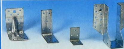
Vinkelbeslag förstärkt används till förband av korsande balkar, vid tyngre konstruktioner. Mått 90x90x2,5 bredd 65 mm. Nr 31-1692 ..... Pris 6:50
