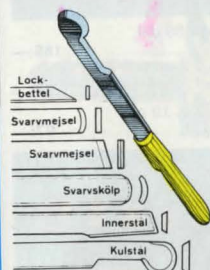
Svarvjärn med skaft av björk, för träsvärning. Längd ca 40 cm.
