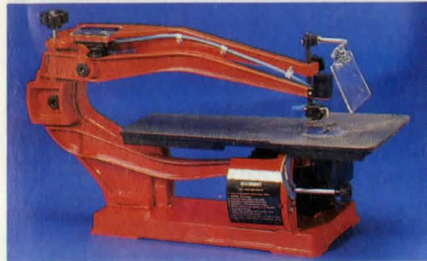
Kontursåg. Kraftig gjutjärnskonstruktion. Hög matningskapacitet. Bordet ställbart 0-45°. Inbyggd spånblåsning. Max såghöjd 50 mm, sågdjup 450 mm. Bladlängd 125-130 mm. (Se lövsågsblad i katalogen). Bladets hastighet 1 720 slag/min. Motor 220 V/95 W. Nettovikt ca 27,5 kg. Nr 40-3558 ..... 1495:—
