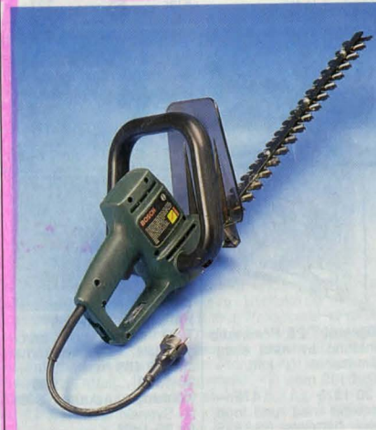
El-häcktrimmer Bosch PHS 46 G. "universalsaxen" med snittlängd 46 cm, 380 W-motor. Ansluts till 220 V. Vikt 3 kg. Max. 13,5 mm. kvistjocklek. Nr 40-3186 ..... Pris 695:—
