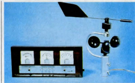
Väder-station för montering utomhus. Inne visar instrument: vindriktning, vindhastighet (två mätområden: 0–10 m/s, 0–45 m/s), inomhustemperatur, utomhustemperatur (-30°–+50°C) samt lufttryck (Bar). Levereras komplett med mätbel och instrumentpanel med 18×41 cm ädelträram samt ca 20 m förbindelsekabel. Drives med ett batteri 32-2212. Nr 34-825 ..... Pris 2290:—
