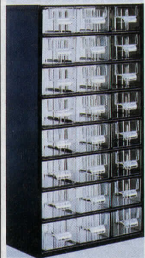
Skåp. Storlek 555×307×146 mm. Med 48 lådor. Vikt 5 kg. Nr 40-1910 ..... 255:—
