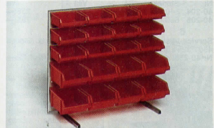
Raaco plockbackar av kraftig plast med stadigt plåtstativ för bord. Kan också hängas på vägg. 12 backar storlek 125×130×50 mm och 8 backar storlek 125×170×75 mm. Vägglåda 520×460 mm. Nr 40-1694 ..... Pris komplett 268:—
