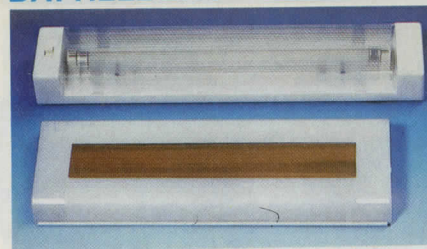
Lysrörsarmatur , med 8 W lysrör. Storlek 368×65×40 mm. 12 V. Reservrör 35-905. Nr 35-936 ..... Pr st 59:—, 10 st 495:—
