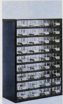
Skåp. Storlek 420×307×146 mm. Med 36 lådor. Vikt 3,9 kg. Nr 40-1904 ..... 205:—
