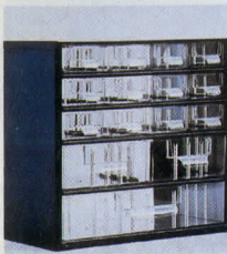
Skåp. Storlek 285×307×146 mm. Med 15 lådor. Vikt 2,5 kg. Nr 40-1903 ..... 155:—
