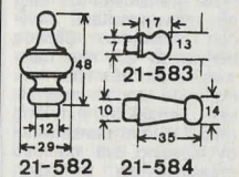
21-582 21-584 Dekorknopp av furu. Nr Pr 2 st 10 st 21-582 7:50 29:—
