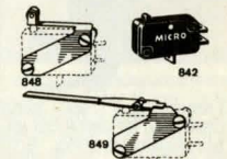
Mikroströmbrytare för 1-polig växling. Honeywell-typ V3-1, brytförmåga likström 0,5 A/125 V växelström 10 A/250 V. I plastkapsel storlek 27x15x10 mm. Nr Pr st 10 st 22-842 6:50 44:-
