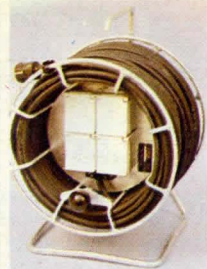
Kabelvinda ELO TYP 750 med 50 m 3x1,5 mm² kabel REVE eller RDOE (oljaresiständig). Av robust förzinkad stålkonstruktion. 4 jordade uttag med sköjtäta lock. Godkänd för utomhusbruk (RDOE även godk. för husvagnar). Kan belastas med 10 A (även hoprullad). Nr Typ Pris 42-1954 REVE 645:- 42-1955 RDOE 720:-
