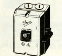
Strömställare plastkapslad. 3-polig strömbrytare. 16 A 380 V. Läsbar i från- och tilläge. Försedd med separat 0-plint. Sköjtät kapsling. 2 genomgående utlopp 22,5 mm. Röd indikatorlampan. Storlek 120x80 mm. Nr 32-1555 ..... 92:-
