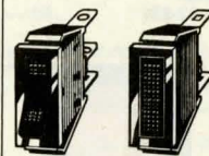
Strömbrytare , 1-polig med inbyggd signallampa. 220 V/10 A. Vit med röd lens. S-märkt. 28x11 mm. Nr Pr st 10 st 22-821 9:50 82:-
