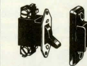
Strömbrytare , 1-polig. 250 V, 6 A. S-märkt. Nr Pr st 10 st 22-2013 8:- 68:-
