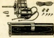
Modellplanmotor L 184 för batterier. (4 st. T 431.) Med skruvar och festsättningsbleck för såväl motor som batterihållare, vilken också har strömbrytare. Propelleraxel ca 3 mm diam. Spinner medföljer. Varvtal med 9 1/2 propeller 1400—1600 varv/min. Propellern frikopplas då den ej drar. Total vikt med batterier och propeller: 135 gram. Utan batterier och propeller 7: 50
