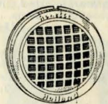
Mikrofonelement M 334. Krystallsystem RONETTE i hölje av plast, storl. 54x16 mm. Frekvensomfång 30—13000. Känslighet vid 1000 p/s, 1,1 mV/μB. Egenkapacitet 2200 pF. Lämpligt belastningsmotstånd 3—10 Mohm. 22: 90
