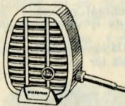
Krystallmikrofon T 937, lämplig för tal. Frekvensområde 100—8000 p/s. Känslighet — 52 dB. Kraftigt plasthölje, storl. 3x6x7,5 cm. Med ca 1 1/2 m skärmsladd. 17: 25
