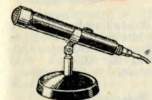
Mikrofon M 470. Högkänslig och formskön dynamisk mikrofon, längd 19 cm. Stabil konstruerad och elegant utförd. Den levereras med ett tungt och stadigt bordsstativ, men lossas lätt för händerdigt bruk som handmikrofon. Impedans 50 K ohm. Känslighet — 70 dB. Omfång upp till över 10.000 p/s. Inbyggd strömbrytare. Med sladd. 55:—
