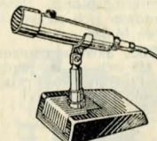
Krystallmikrofon M 471. Behandlad handmikrofon i stavmodell av förkromad metall, längd 13 cm. Med strömbrytare, sladd och löstagbart bordsstativ. Frekvensområde 150—8.000 p/s. Känslighet — 63 dB. 29:—
