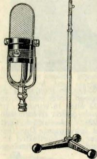
Mikrofon M 597, högkänslig bandmikrofon. Finnes för 600 Ohm eller 30 KOhm. Känsligheten är — 75 dB vid 600 Ohm. Frekvensområde 40—10000 Hz. Mycket användbar för HI—FI utrustningar o. överallt där hög känslighet och hög kvalitet efterfrågas. Fint högljansförmickad och försedd med fäste för montering på stativ. 167:—
