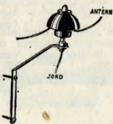
Åskskydd T 1259 för TV-nedledning (band- eller slangkabel). Fäste för montering på vägg. Skyddet sitter 10 cm från väggen. Nedledningen dras genom skyddet, och detta jordas med kopparring; exp.-vis N 441. 3: 10
