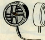
Mikrofon M 598, kolkornskapsel av högsta kvalitet. Impedans 10 Ohm. Känslighet — 46 dB vid 1000 Hz. Diam.: 4 cm. Med 1 m lång, skärmd kabel. 6: 90
