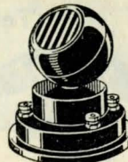
Mikrofon M 573. Kolkpulvermikrofon med inbyggd transformator. Hölje och fot av pressad bakelit. En liten trevlig mikrofon, för anslutning till grammofoonuttaget på radioapparater. Matas med vanl. ficklampsbatterier. 14: 20
