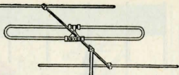
TV-antenn T 782 av 10 mm aluminiumrör. Dipol med reflektor och direktor samt mastfäste. För 240—300 ohms anslutningskabel. 6,5 dB. Riktiv. 7:1. För kanal 5, 6, 7, 8, 9, 10 eller 11. 24:—
