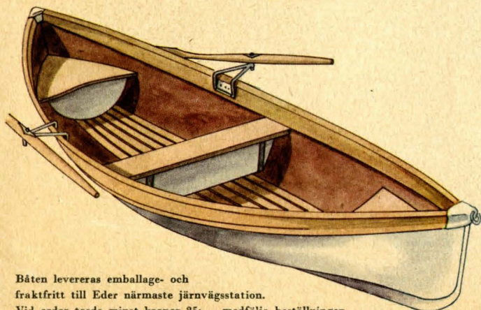
Tre inbyggda vattentäta skott gör båten osänkbar
