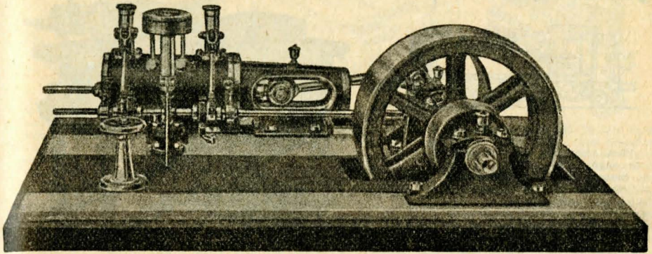
Ventilångmaskin RD 115.
