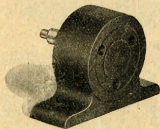
Kopplingsplint № T109, för anslutning av antenn och jordledning till apparaten vilket sker med vanliga bananstift. Plinten fästes på bottenplattan inuti apparaten, och för bananstiften borras hål i radiolådans baksida. Praktisk och prydlig. Pris pr st. . . . . 1.80
