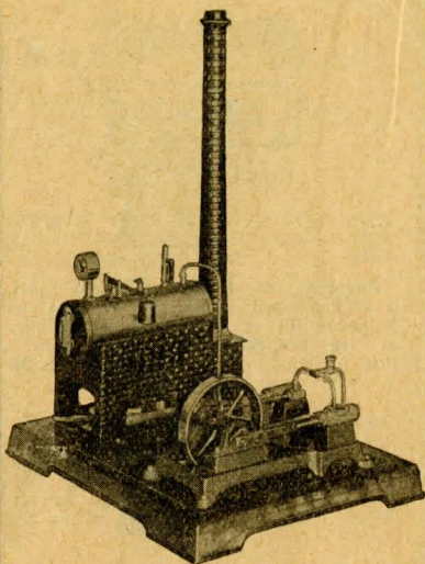
Ångmaskin № L 22, med liggande stor ångpanna av oxiderad mässingplåt, två stycken dubbelverkande fasta cylindrar monterade på järnsoclel, manometer som visar ångtrycket, ångvissla, vattenståndsrör, förnicklat och lackerat balanshjul. En mycket elegant och solid maskin. Bottenplattans storlek 23x28 cm. Höjd med skorsten 39 cm. Maskinen går såväl fram som back. Pris . . . . . 21.50
