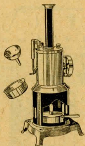
Ångmaskin № L 20, med ångpanna av fjock, polerad mässingplåt, rörlig mässingscylinder. Eldas med sprit. Tratt, vattenmått och spritlampa medföljer. Höjd med skorsten 24½ cm. Pris . . . 2.50
