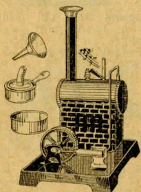
Ångmaskin № L 21, med liggande ångpanna av oxiderad mässingplåt, rörlig cylinder av förnicklad mässing, vissepipa, säkerhetsventil, tratt, spritlampa och vattenmått. Bottenplattans storlek 16½x12 cm. Pris . . . . . 4.90
